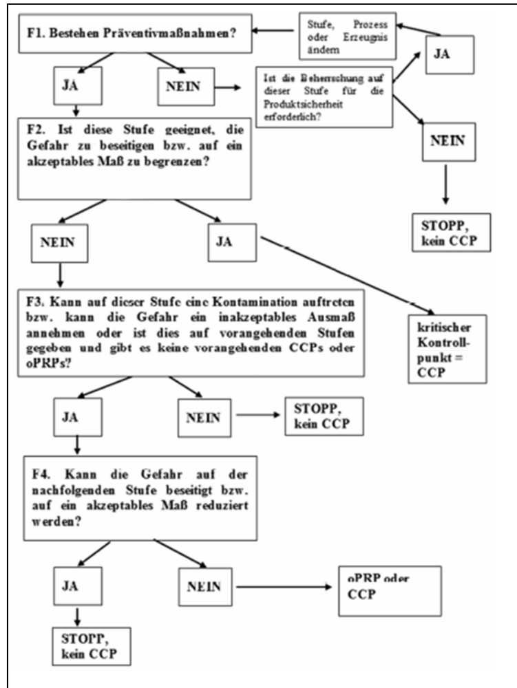
Abbildung 1: Entscheidungsbaum zur Bestimmung von CCPs (Quelle: (Europäische Kommission 2016, Seite 29))
